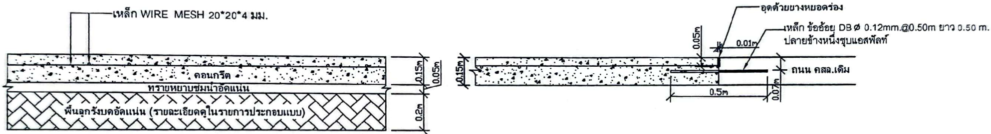
รายละเอียดถนนคอนกรีตเสริมเหล็ก
