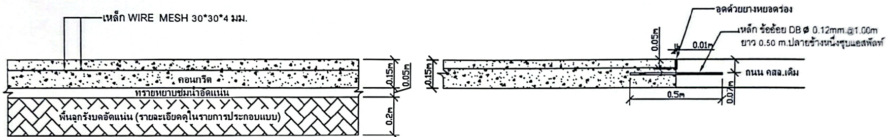
รายละเอียดถนนคอนกรีตเสริมเหล็ก
